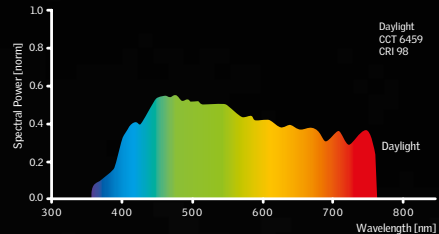
Tageslichtkurve
