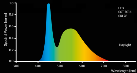
Kurve einer elektrischen LED-Lichtquelle
