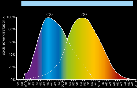
Durch Licht ausgelöste Reaktion des zirkadianen (C( \lambda )) und des visuellen (V( \lambda )) Systems (Pechacek et al., 2008)
