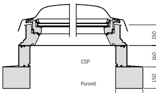
Finestre per tetti piani CSP EFC con telaio di estensione fisso. Con telaio di estensione aggiuntiva in Purenit
